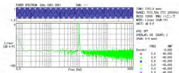
周波数分析(FFTグラフ)
